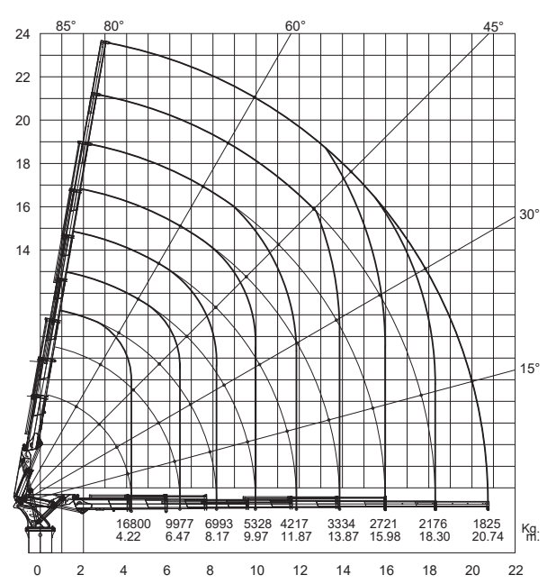
25 Ton ASK 75 TM Gemi Vinci / Marine Cranes
